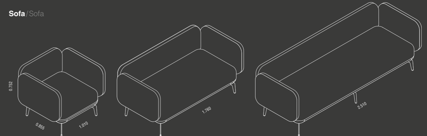
Sofa mit Umhausung / Sofa with Casing
